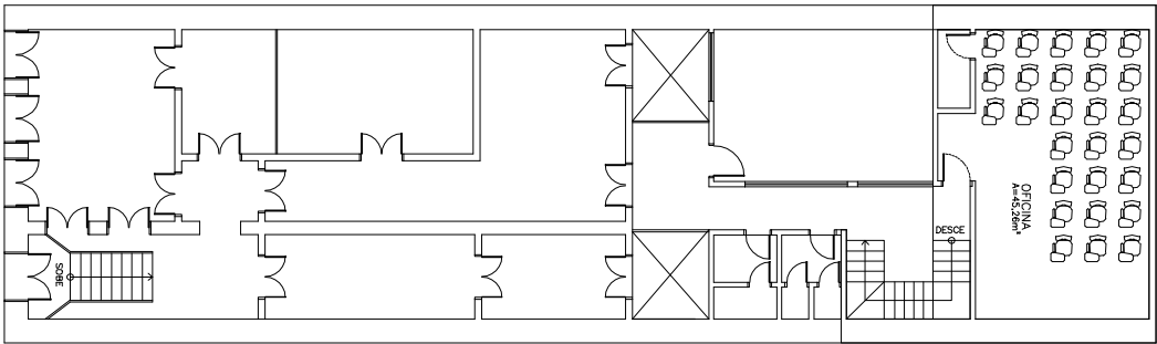
PLANTA BAIXA PAV SUPERIOR ESCALA — 1 : 75
