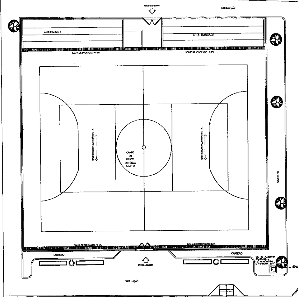
PLANTA BAIXA TÉRREO ESCALA: 1/75
