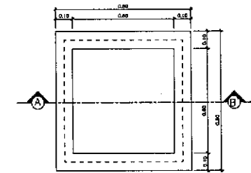
PLANTA BAIXA
