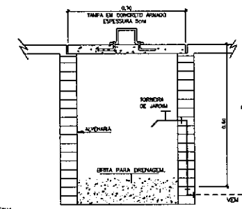
CORTE - A B'
