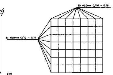
FERRAGEM DA TAMPA
