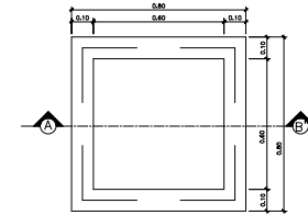
PLANTA BAIXA
