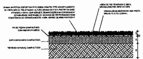
DETALHE DISPOSIÇÃO GRAMADO SINTÉTICO S/ ESCALA
