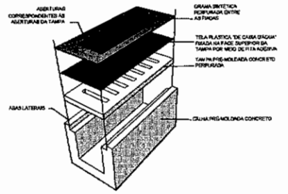
DETALHE CANALETA LATERAL S/ ESCALA
