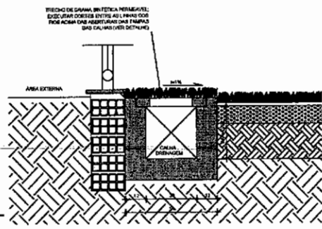
DETALHE CANALETA LATERAL S/ ESCALA
