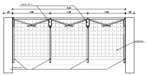
CORTE C ESC.: 1:20
