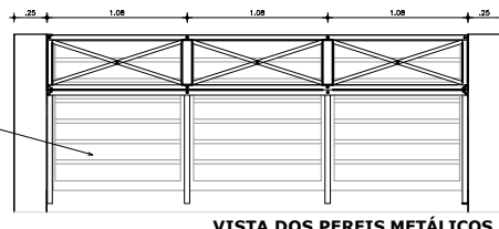
VISTA DOS PERFIS METÁLICOS ESC.: 1:20
