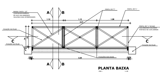
PLANTA BAIXA ESC.: 1:20
