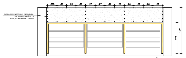
VISTA DA PLACA CIMENTÍCIA ESC.: 1:20
