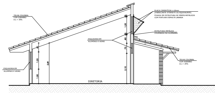
CORTE - D ESC.: 1:50
