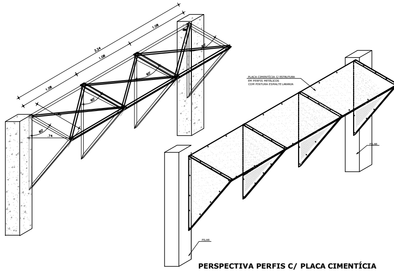
PERSPECTIVA PERFIS C/ PLACA CIMENTÍCIA ESC.: 1:20
