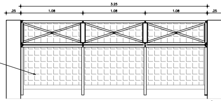
VISTA DOS COMBOGÓS ESC.: 1:20
