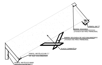
DETALHE SOBREPOSIÇÃO DE PEÇAS ESC.: 1:10
