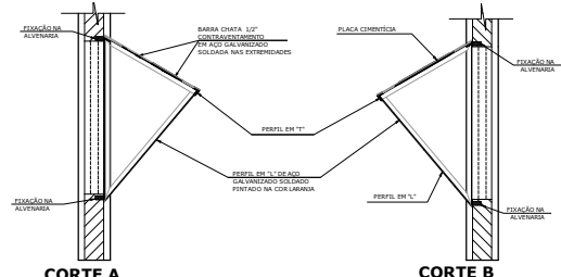
CORTE A ESC.: 1:20
