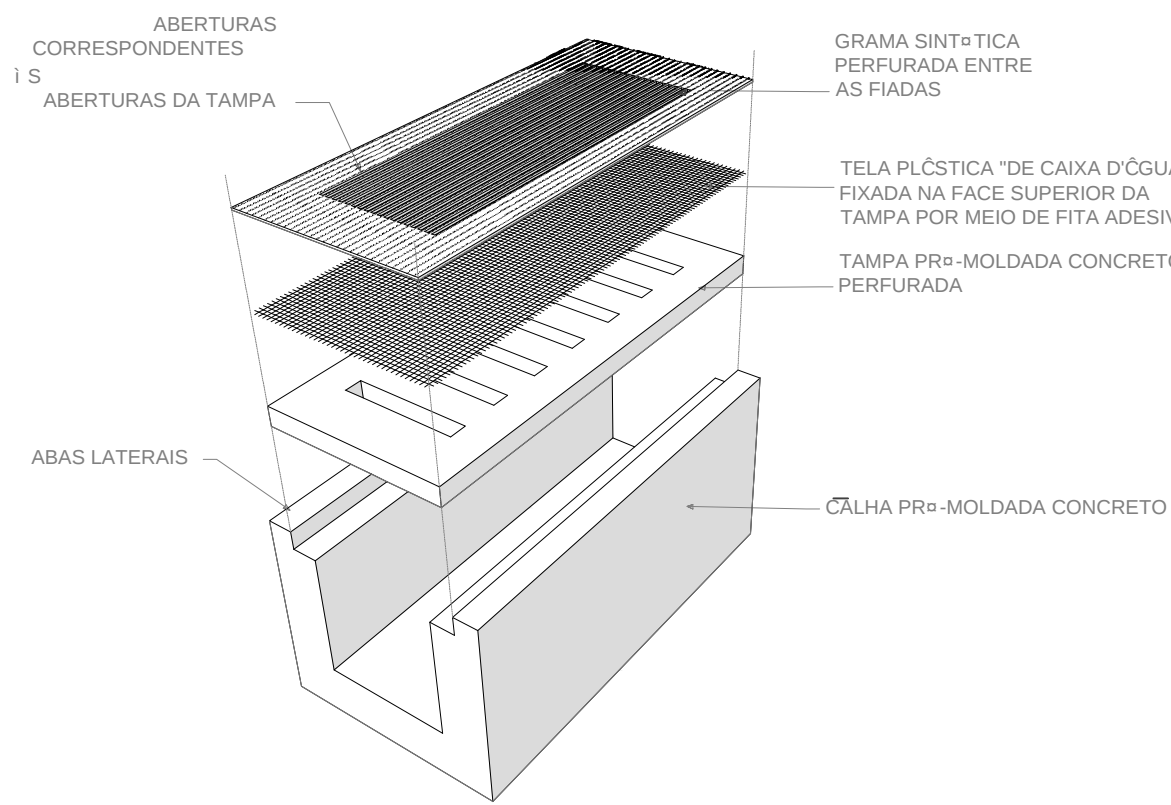
DETALHE CANALETA LATERAL S/ ESCALA
