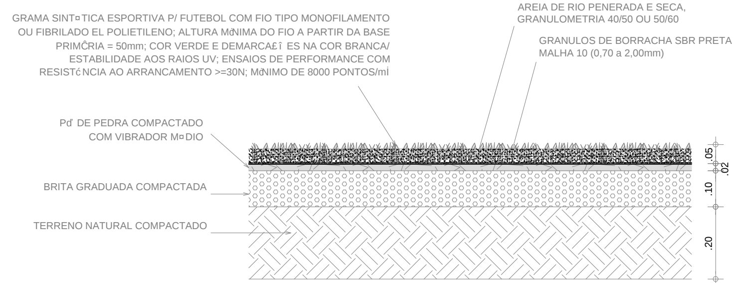
DETALHE DISPOSIÇÃO GRAMADO SINTÉTICO S/ ESCALA
