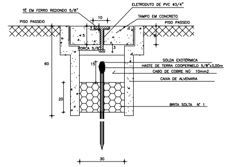
DETALHE ATERRAMENTO SEM ESCALA
