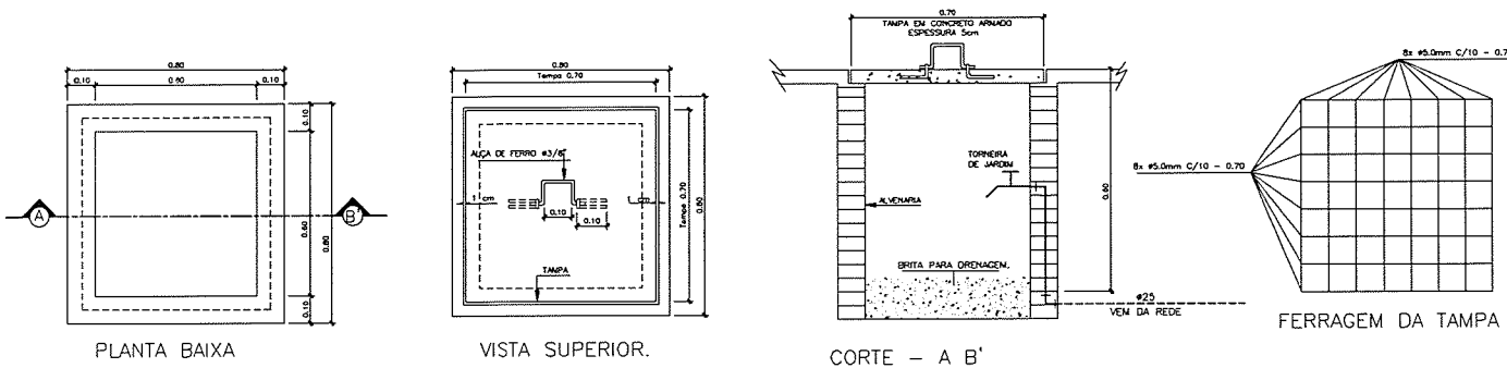
DETALHE EXECUTIVO DA CAIXA COM TORNEIRA DE JARDIM CAIXA DE PASSAGEM 60x60x60cm - TAMPA DE CONCRETO
