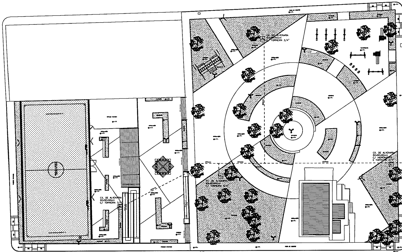
PLANTA BAIXA ESCALA 1/200
