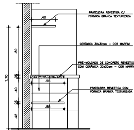
SEÇÃO C - PRATELEIRAS esc. 1:50
