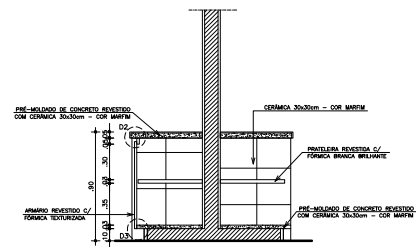
SEÇÃO D - ARMÁRIO AB1/AB2 esc. 1:50
