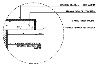
DETALHE D3 esc. 1:5
