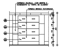
VISTA - GAVETEIRO G2 esc. 1:50
