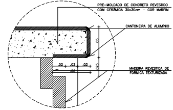
DETALHE D2 esc. 1:5
