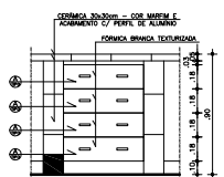
VISTA - GAVETEIRO G1 esc. 1:50
