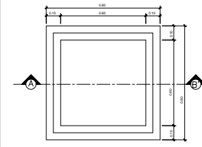
PLANTA BAIXA
