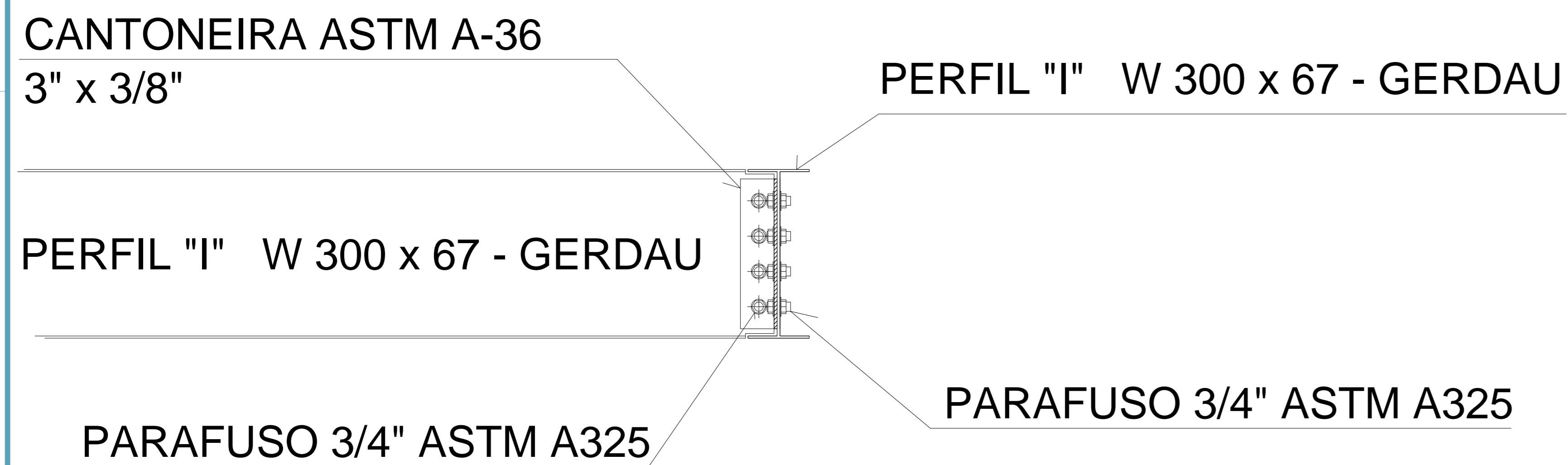
DETALHE 03 escala 1:10
