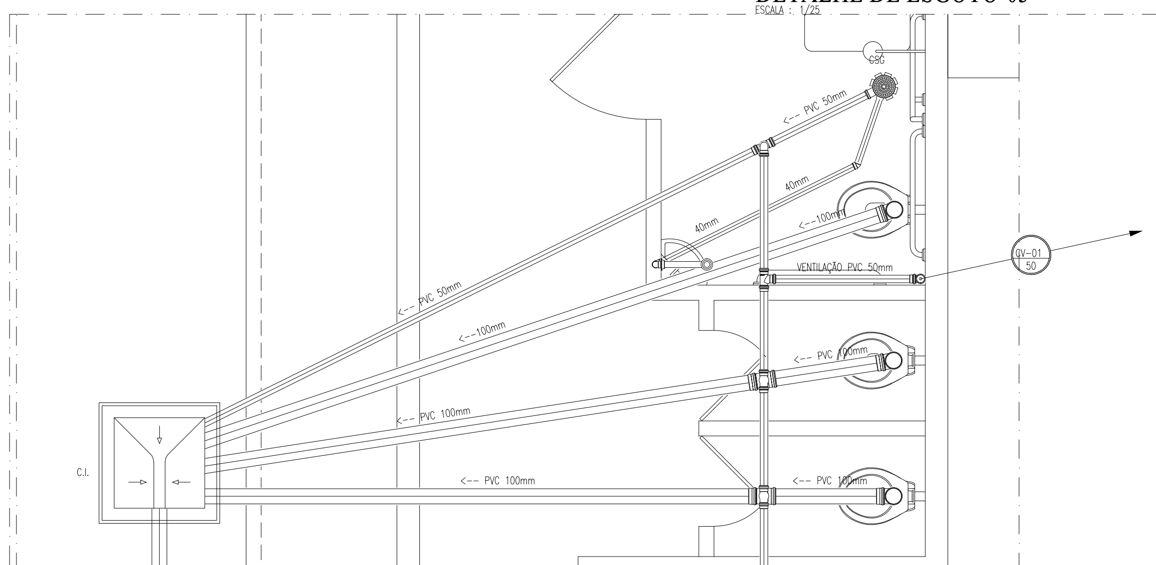
DETALHE DE ESGOTO-01
