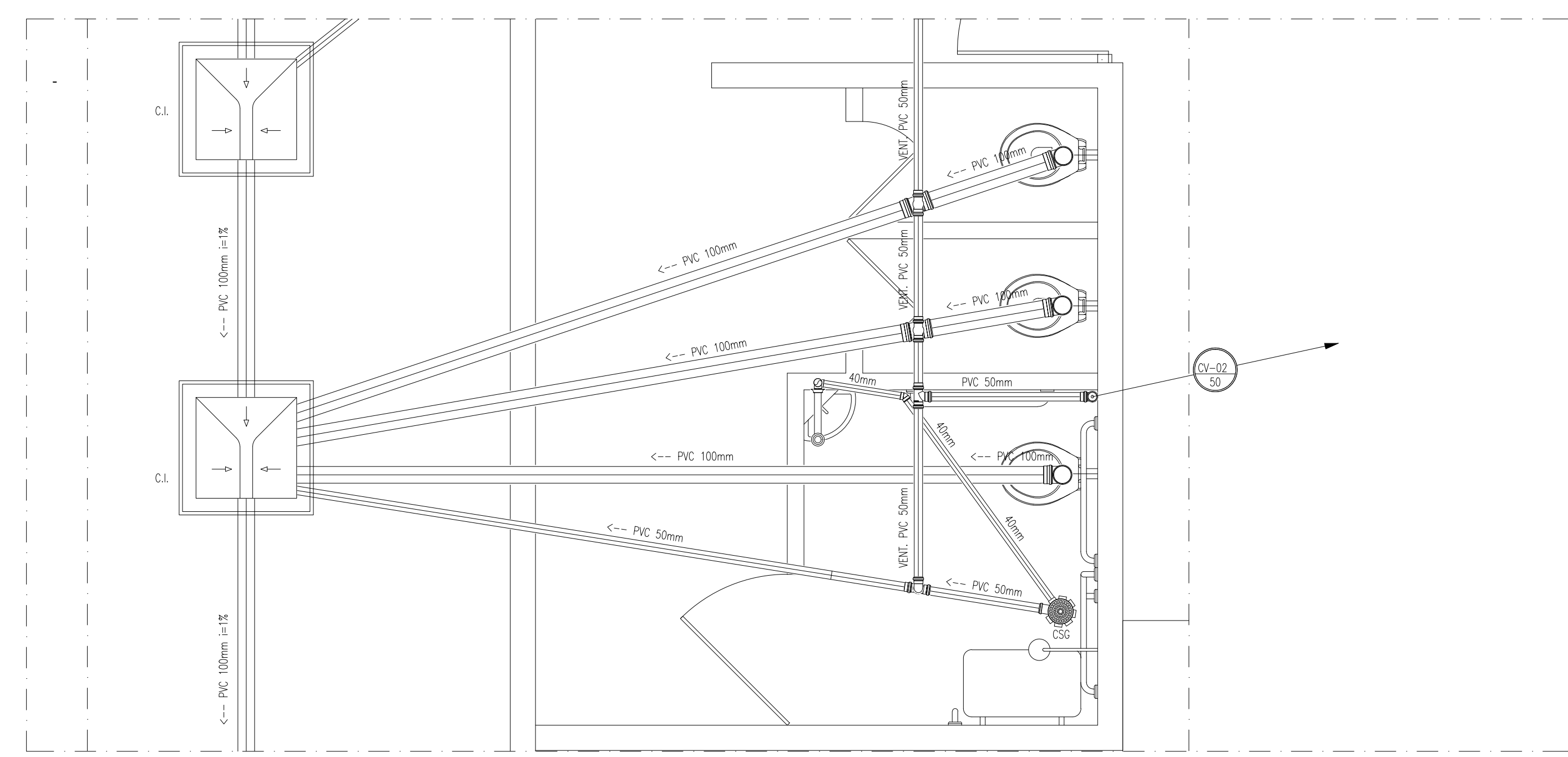
DETALHE DE ESGOTO-04
