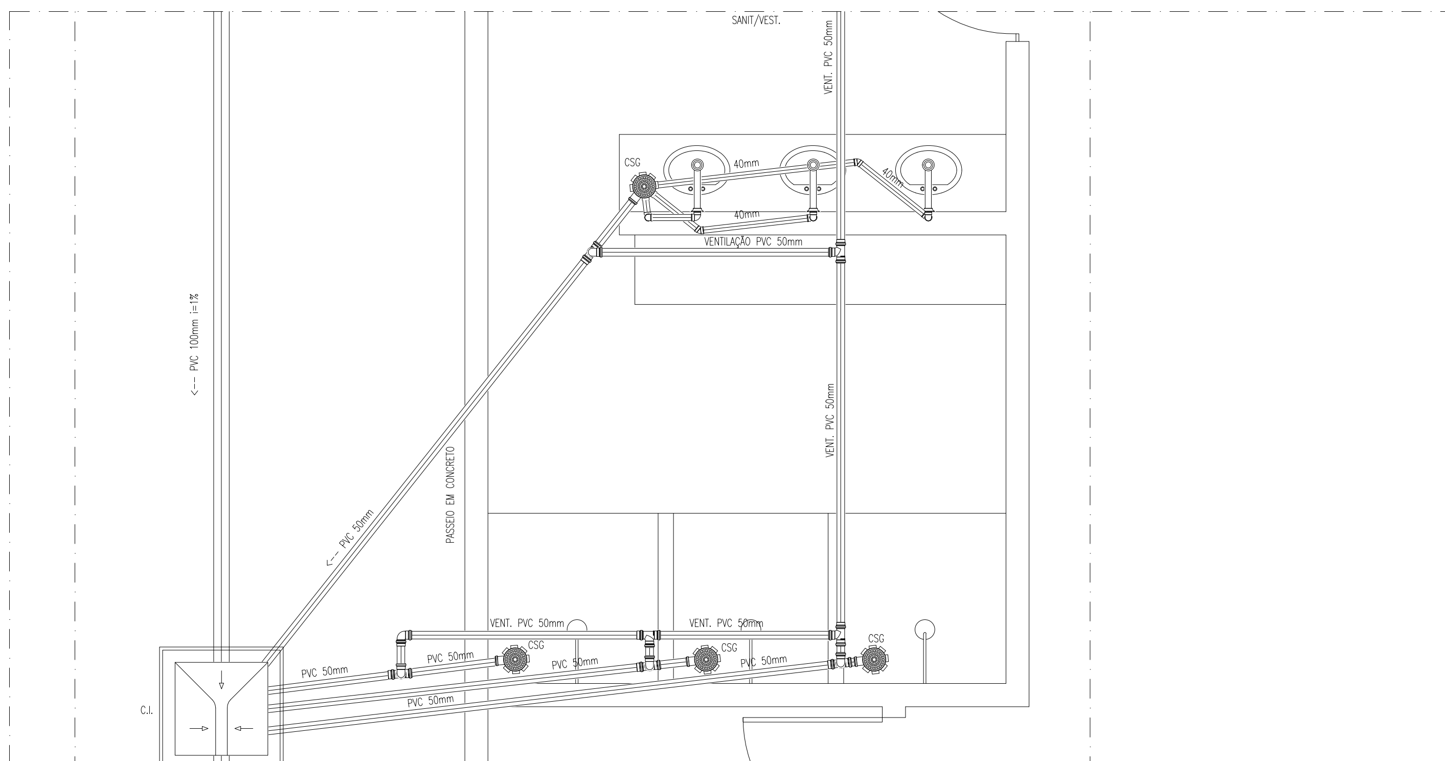
DETALHE DE ESGOTO-02
