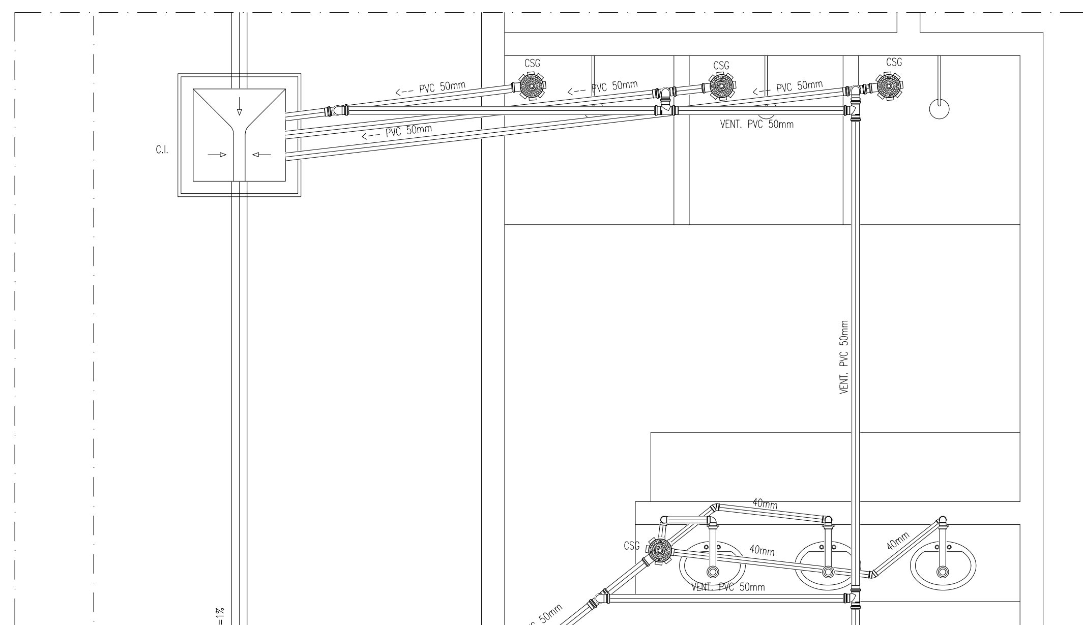
DETALHE DE ESGOTO-03
