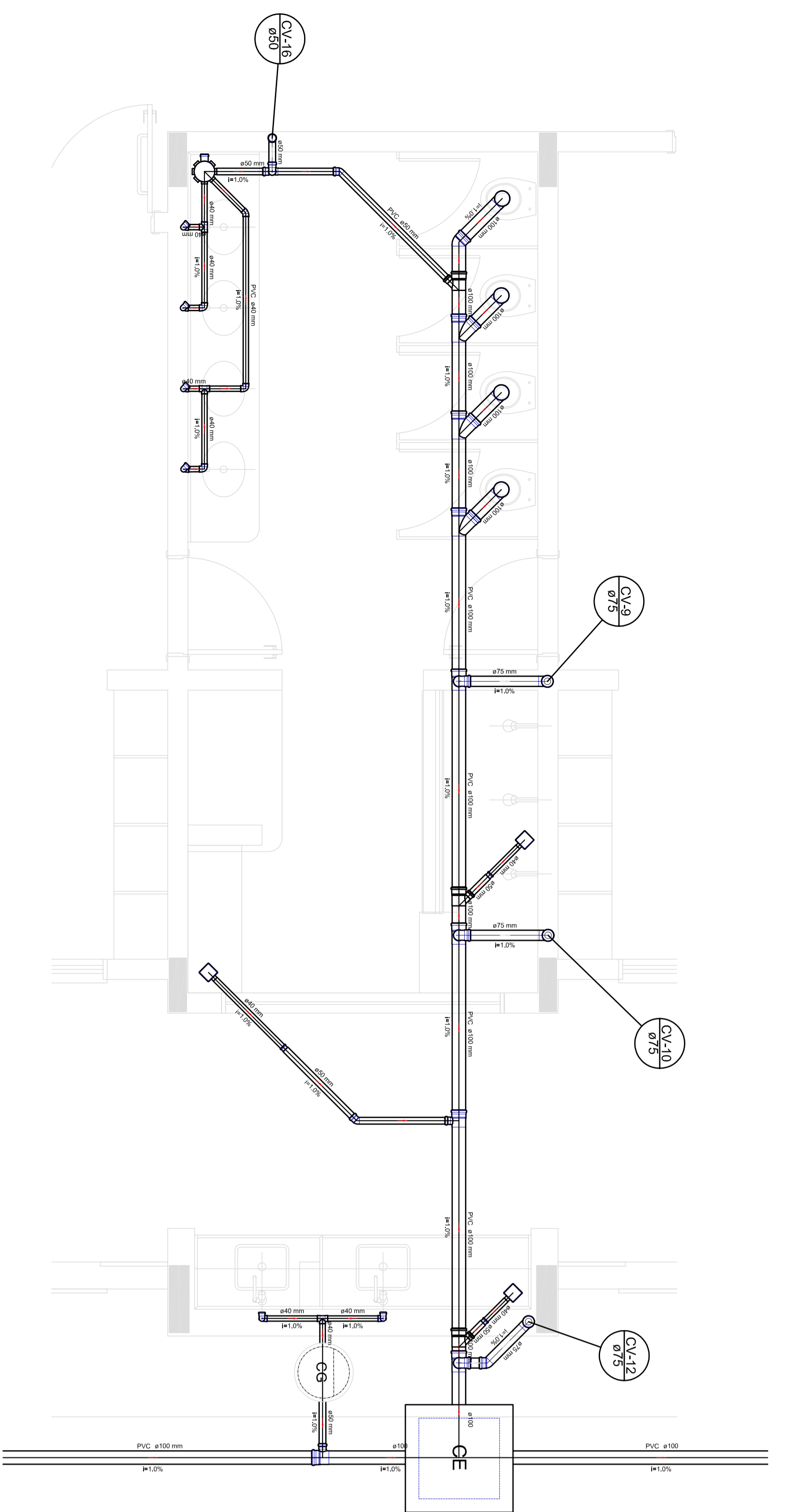
Detalhe S9 escala 1:25
