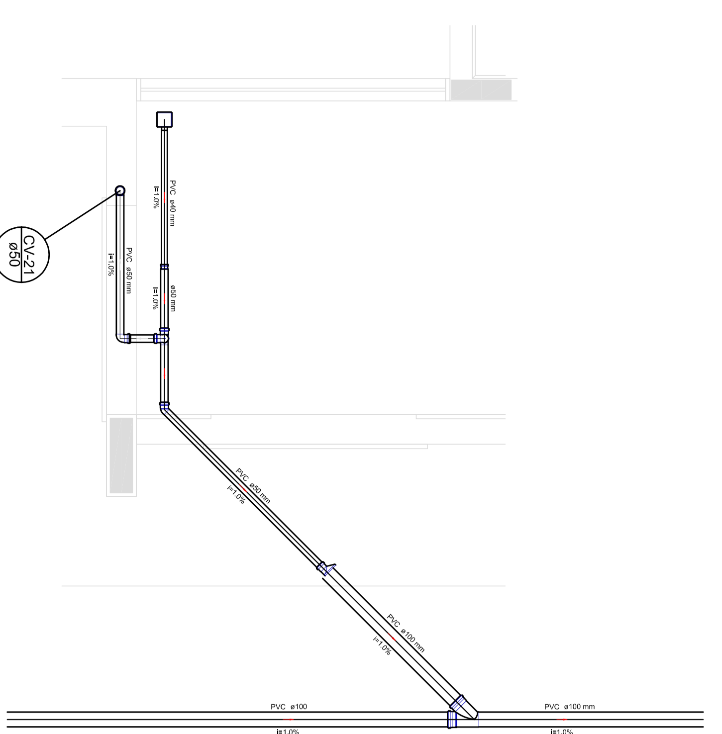
Detalhe S11 escala 1:25
