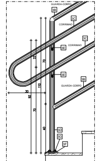
VISTA LATERAL - CORRIMÃO COM GUARDA-CORPO P/ ESCADA ESC.: 1:10
