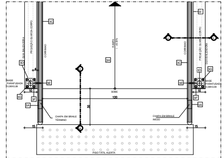
PLANTA BAIXA - CORRIMÃO COM GUARDA-CORPO ESC.: 1:20
