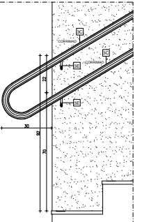
VISTA LATERAL - CORRIMÃO FIXADO EM ALVENARIA - PARA ESCADA ESC.: 1:10
