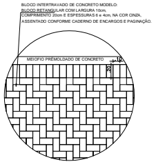
DET. PISO INTERTRAVADO ESC.: 1:25
