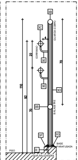
CORTE AA - CORRIMÃO COM GUARDA-CORPO - RAMPA ESC.: 1:10
