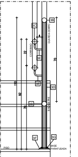
CORTE AA - CORRIMÃO COM GUARDA-CORPO P/ ESCADA ESC.: 1:10
