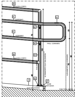
VISTA LATERAL - CORRIMÃO COM GUARDA-CORPO - RAMPA ESC.: 1:10
