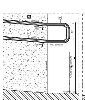
VISTA LATERAL - CORRIMÃO FIXADO EM ALVENARIA - RAMPA ESC.: 1:10
