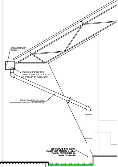
DET. CALHA(QUADRA COBERTA) ESC.: 1:25
