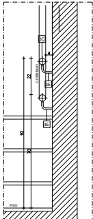
CORTE - CORRIMÃO FIXADO EM ALVENARIA P/ ESCADA ESC.: 1:10
