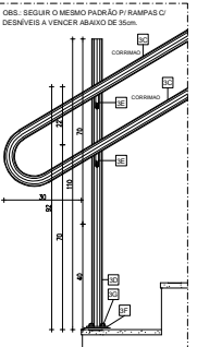
VISTA LATERAL - CORRIMÃO SEM GUARDA-CORPO P/ ESCADA ESC.: 1:10
