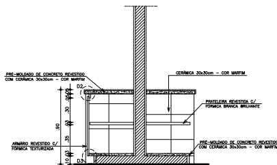
SECÇÃO D - ARMÁRIO AB1/AB2 ESC: 1:20
