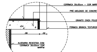
DETALHE D3 ESC: 1:2
