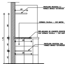
SECÇÃO C - PRATELEIRAS ESC: 1:20
