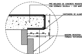
DETALHE D2 ESC: 1:2
