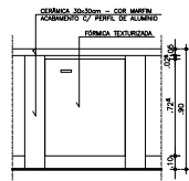
VISTA - ARMÁRIO AB1/AB2 ESC: 1:20
