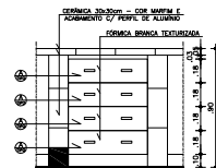
VISTA - GAVETEIRO G1 ESC: 1:20
