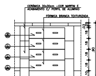
VISTA - GAVETEIRO G2 ESC: 1:20
