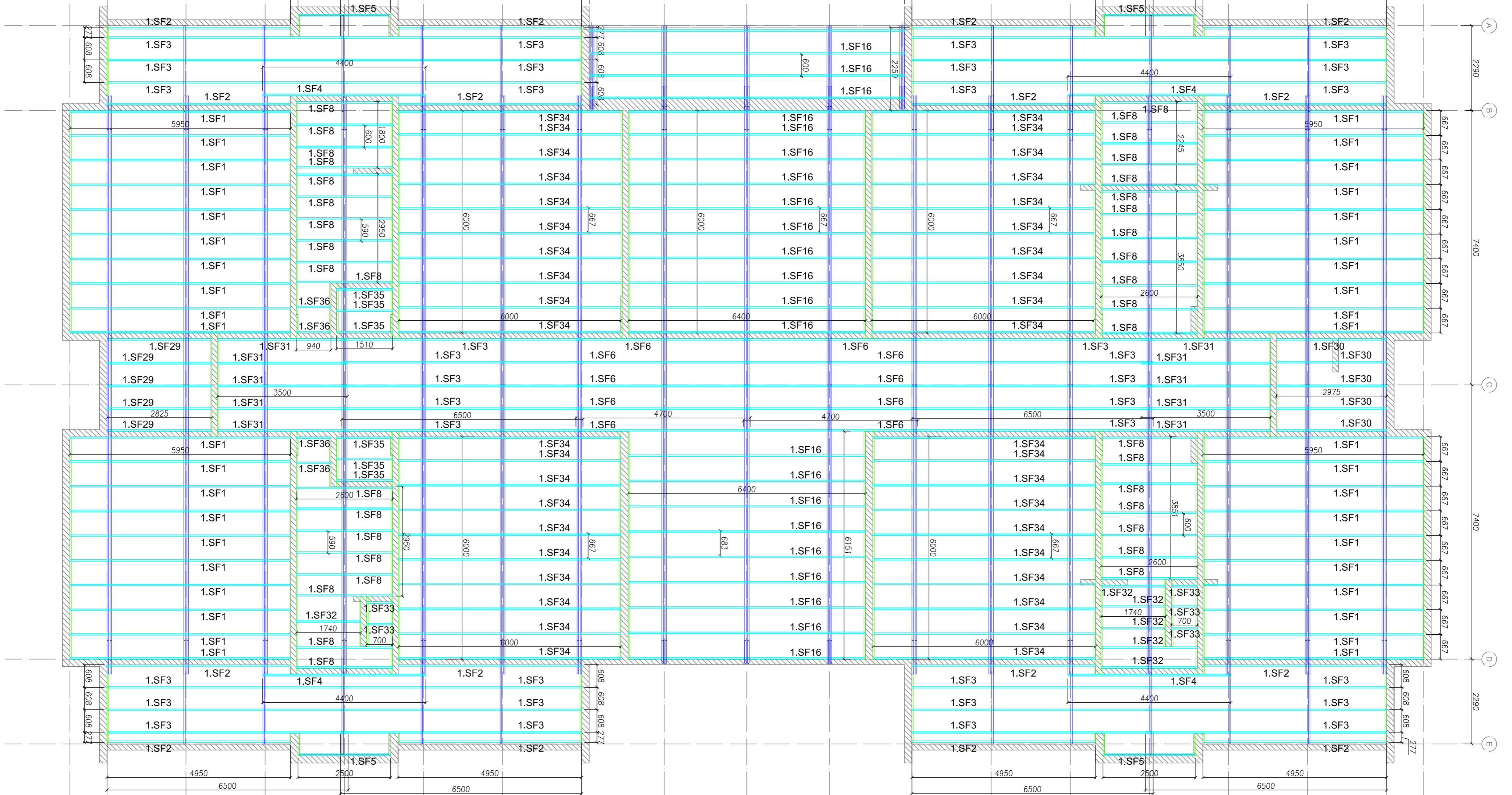
2 BLOCO B - VISTA EM PLANTA - SUPORTES DO FORRO ESCALA: 1/75
