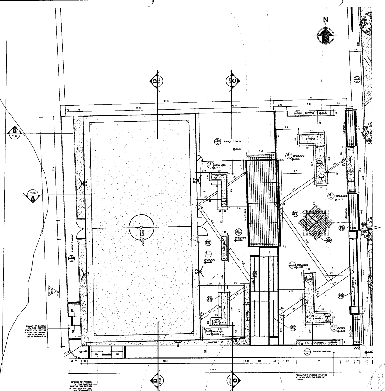
1 Planta de Obra Trecho 02 ESCALA 1/125
